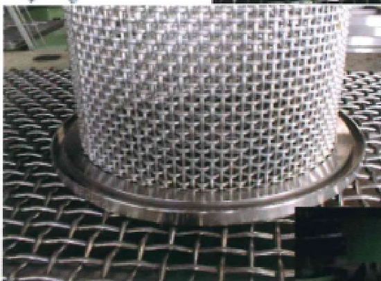
Sonderfilterkorb für Hochdruckanwendungen Maschenweite: 4 mm Draht: 2 mm
