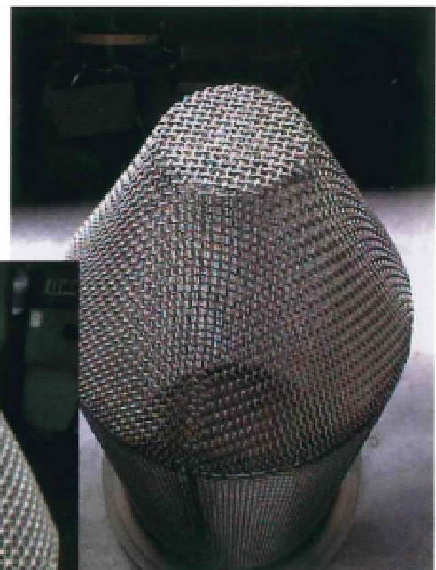
Druckfilterkorb Größe II mit Boden als gezogenem Kegelstumpf
